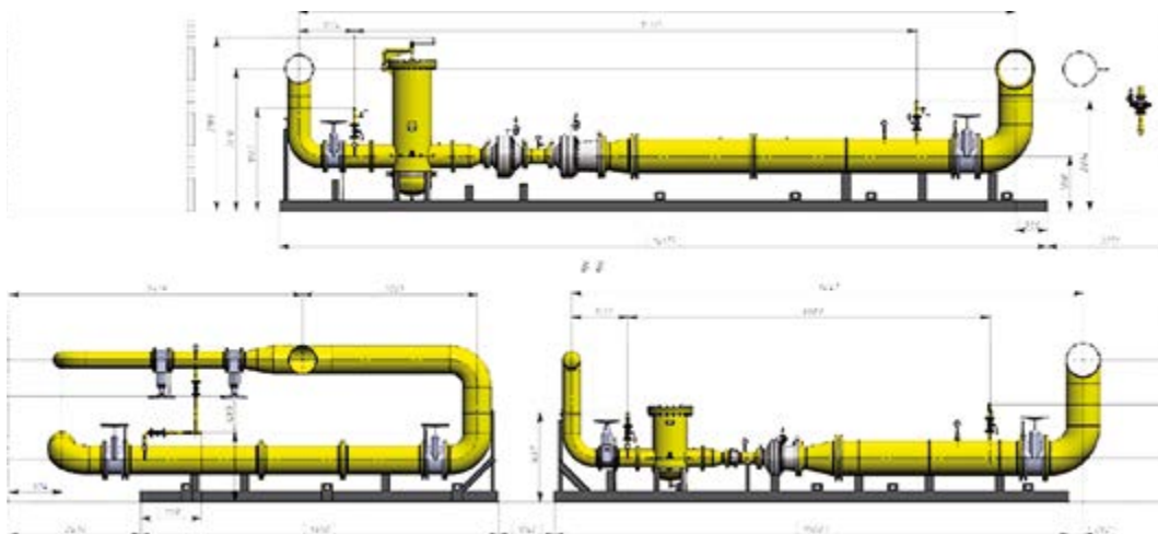
Компоновочное решение для линии редуцирования в составе ГРП
